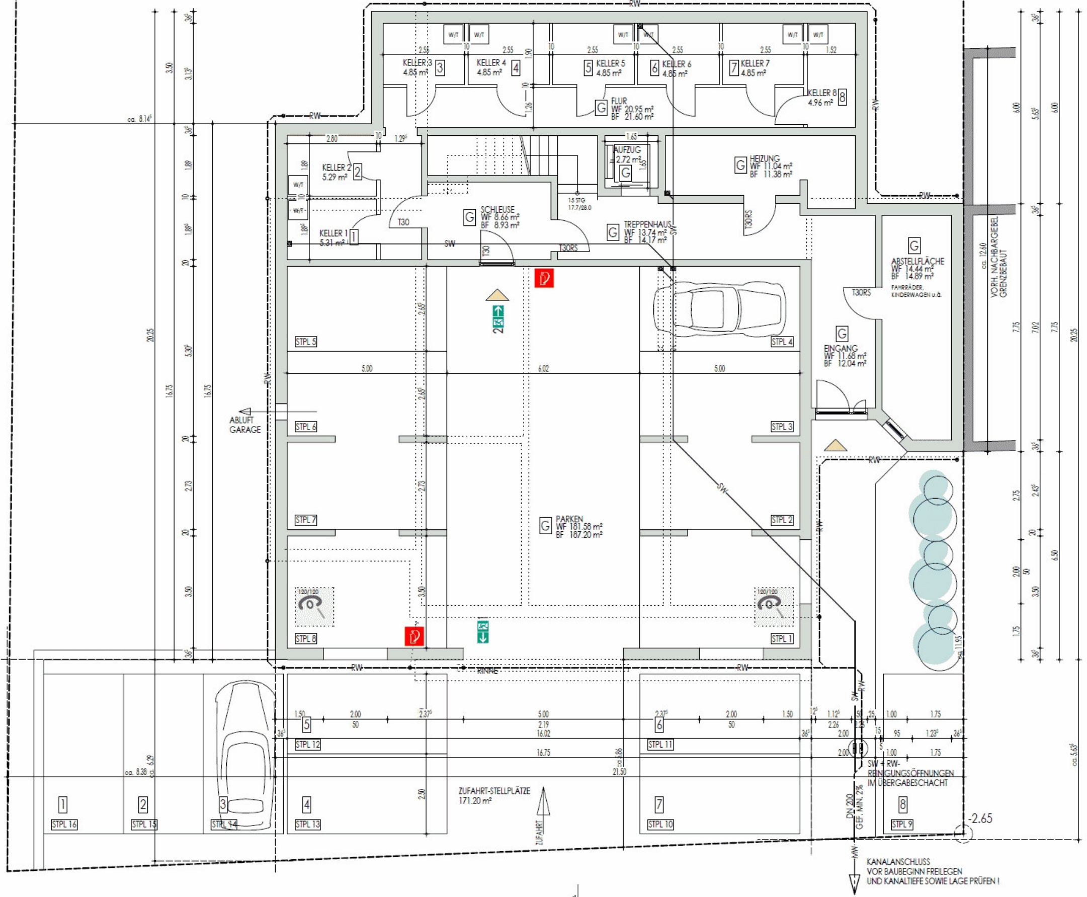
GRUNDRISS KELLERGESCHOSS
