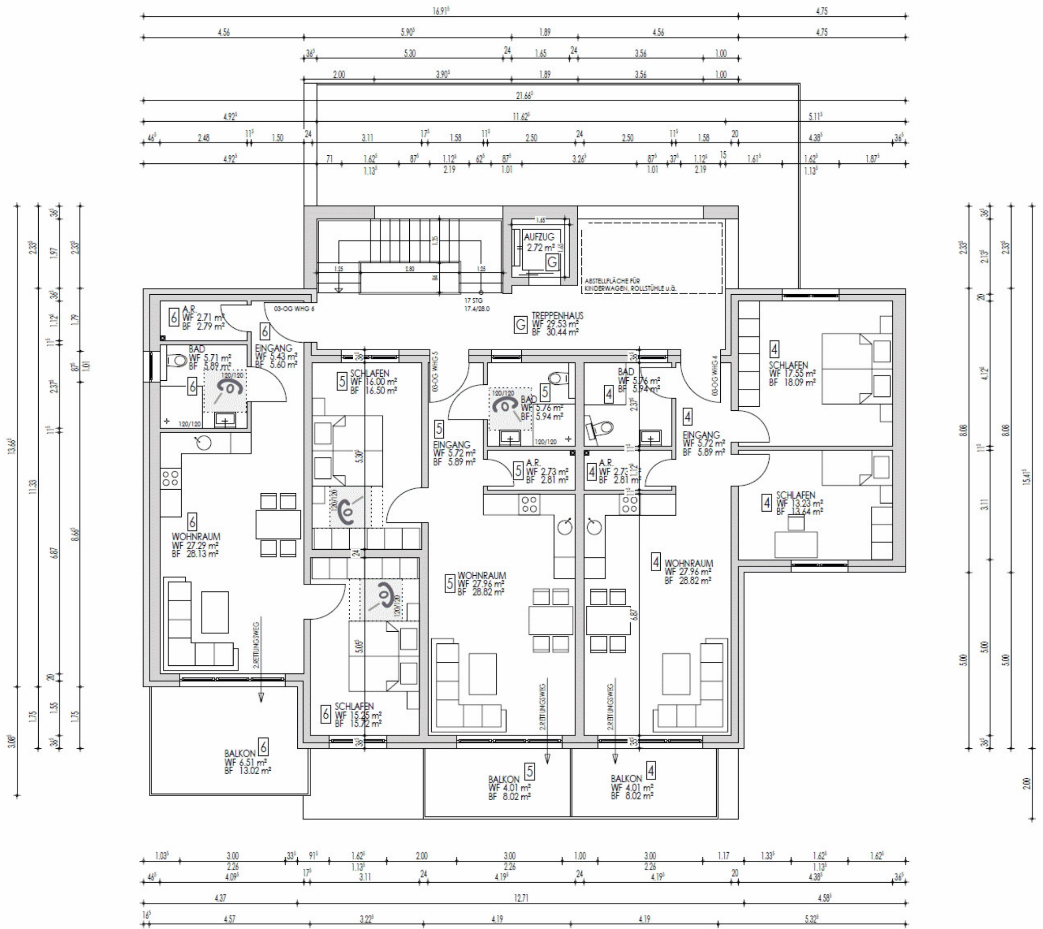
GRUNDRISS OBERGESCHOSS
