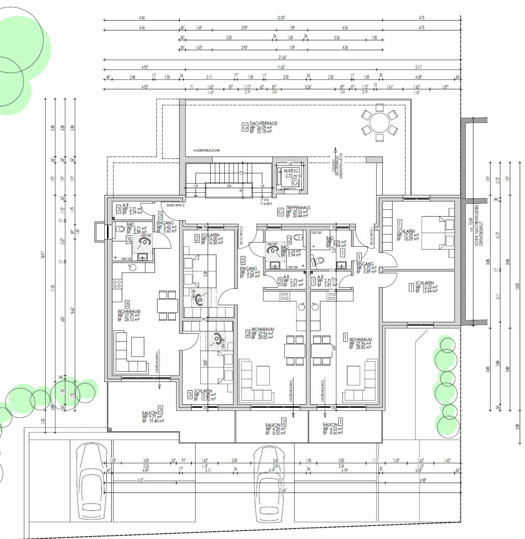
GRUNDRISS ERDGESCHOSS
