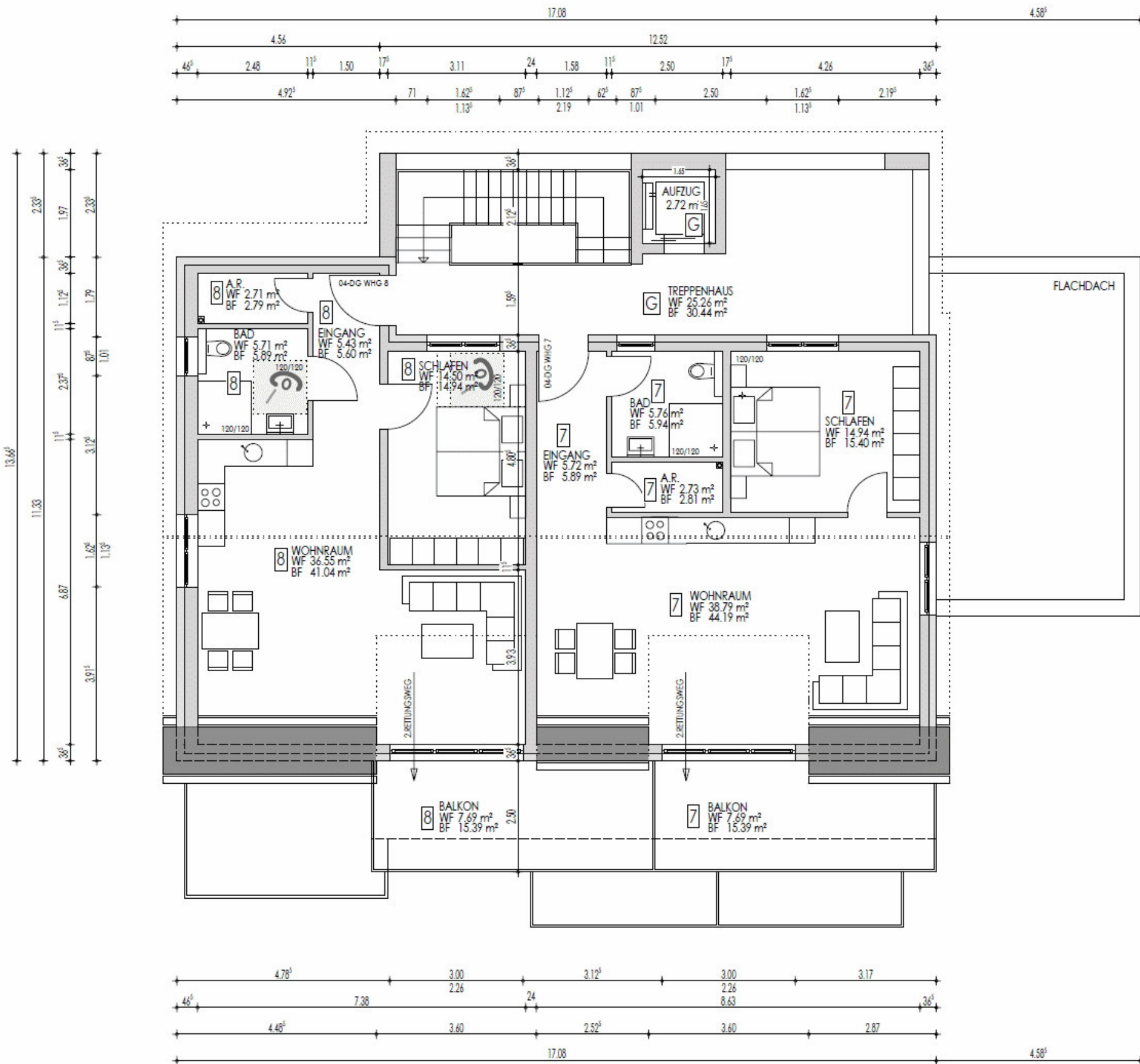
GRUNDRISS DACHGESCHOSS
